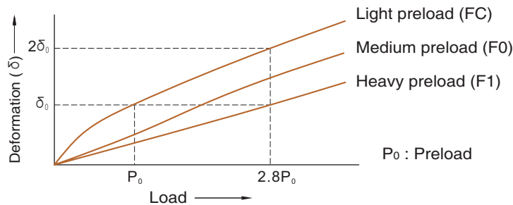
Fig.10 Rigidity
