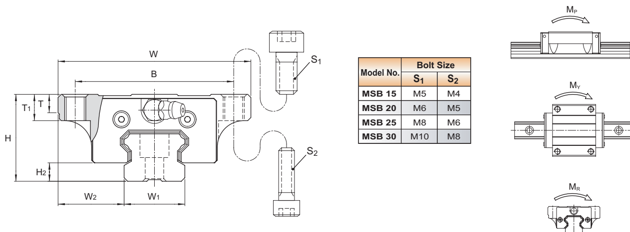
MSB-E
