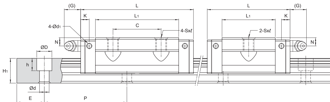
MSB-E
