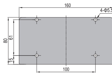
Conduit Cap-80x160
