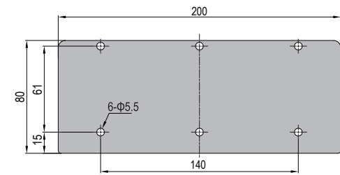
Conduit Cap-80x200
