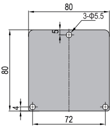
Conduit Cap-80x80
